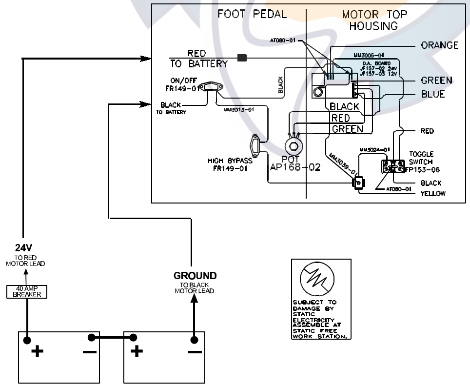
12V & 24V D.A. WIRING DIAGRAM
